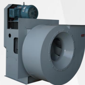
高温插入式离心风机
